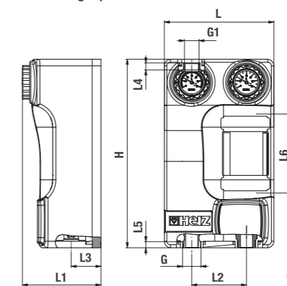
Dimensiones grupos hidráulicos calefacción
