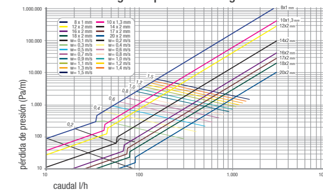
Diagrama pérdida de carga
