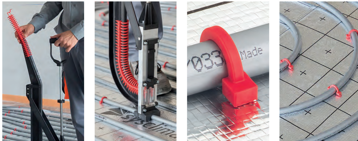
Grapa de fijación Sysclima 3D profesional para tubo Ø 16. Placas aislantes con espesor ≥ 20 mm.
